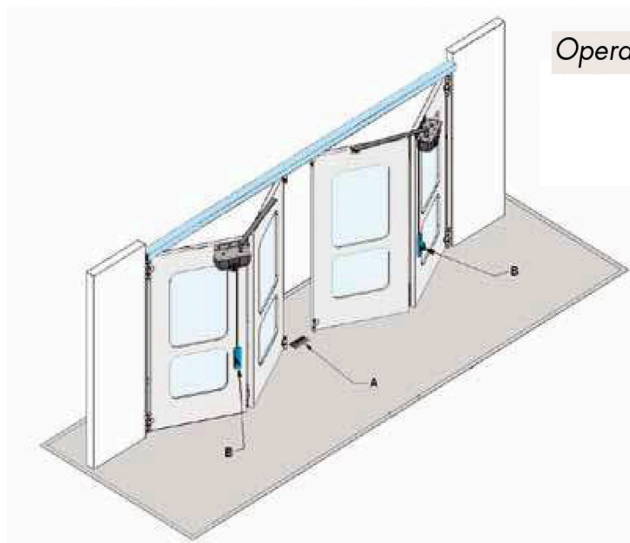
Operador montado en la pared, por encima o por debajo de la guía, abertura posible a más de 120°
