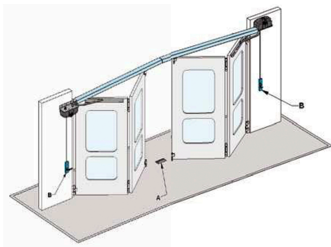
Dos operadores montado en la puerta 4+0 hojas
